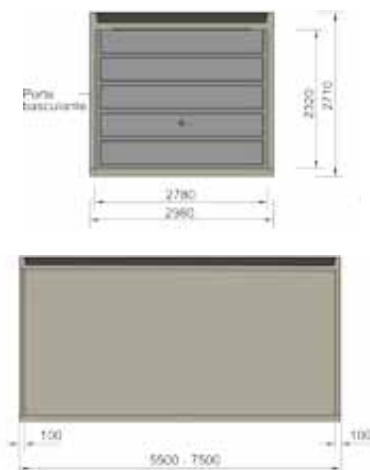
Container simple avec habillage des parois en bois
