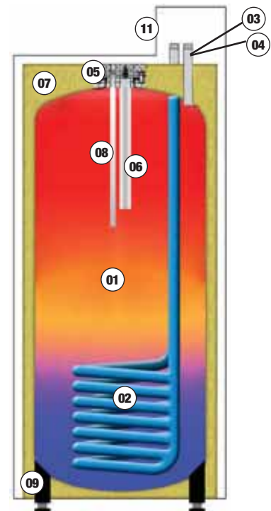
Nano-Ballon 210 litres en coupe
