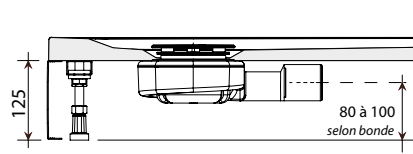
1. Posée sur châssis avec tablier 125 mm
