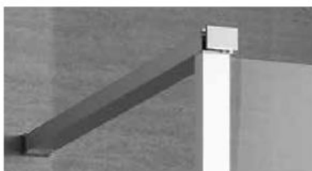
BARRE DE STABILISATION MURALE JAZZ+ DOUCHE OUVERTE avec patère rétractable en bout de barre. Fixation sur le profilé de la paroi / Permet de stabiliser une paroi fixe seule au mur. Pièce de fixation murale et la patère retractable en finition Argent brillant quelle que soit la finition de la barre. Un élément de stabilisation est obligatoire pour une paroi JAZZ+ \geq 800 mm.
