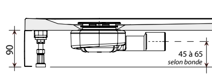
2. Posée sur châssis avec tablier 90 mm
