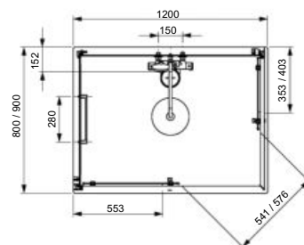
A RECTANGLE 1200x800 et 1200x900
