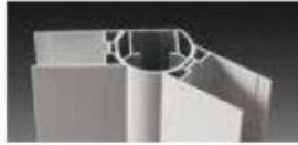
PROFILÉ DE LIAISON ORIENTABLE Permet le montage, en biais, d'une paroi fixe et d'une porte ou de 2 parois fixes DOUCHE OUVERTE jusqu'à 180°.
