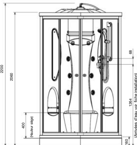
Receveur avec châssis et pieds réglables
