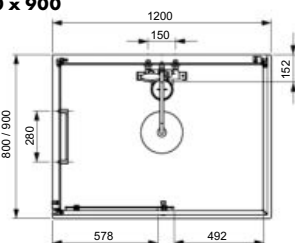
B RECTANGLE 1200 x 800 et 1200 x 900
