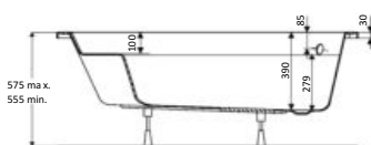
Version gauche 150x 100, 150x85, 145x95, 140x90
