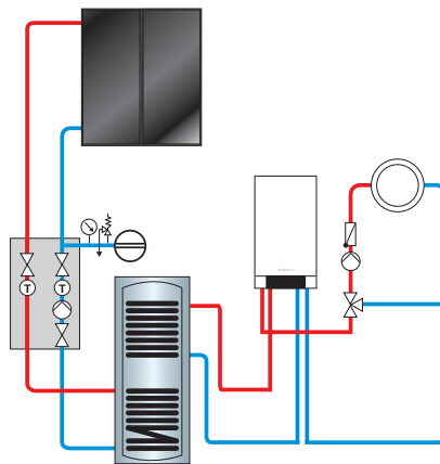
Production d'eau chaude sanitaire solaire
