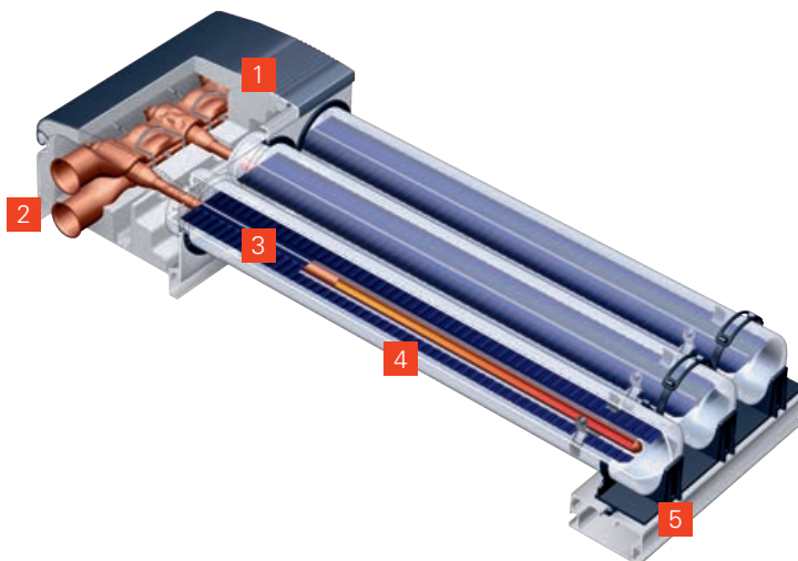
Installation simple et orientation rapide de l'absorbeur grâce à l'indicateur angulaire sur les logements pour tubes
