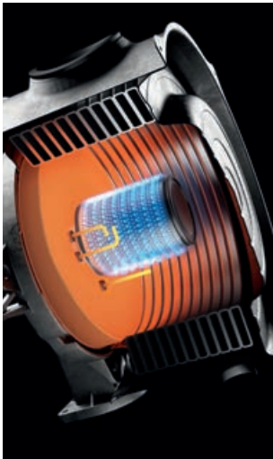
Brûleur MatriX-Plus
