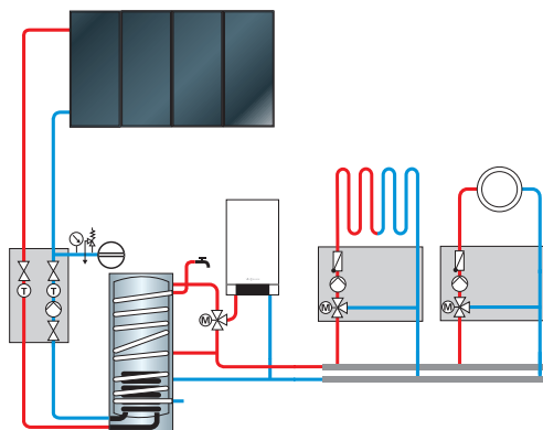
Production d'eau chaude sanitaire solaire et appoint de chauffage solaire
