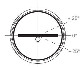
Installation simple et orientation rapide de l'absorbeur grâce à l'indicateur angulaire sur les logements pour tubes
